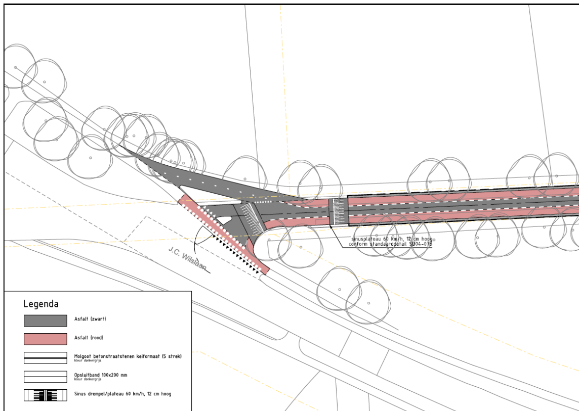
Figuur 1: Wegprofiel met drempel Soerenseweg Figuur 2: Kruispunt Soerenseweg
